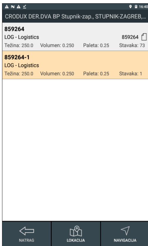
Slika 9. Ekran za pregled i obradu dokumenata dostave
