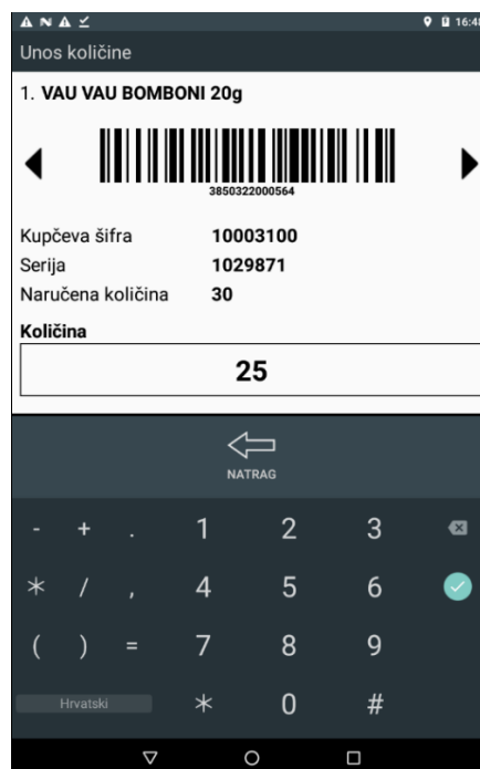
Slika 11. Unos isporučene ili prikupljene količine
